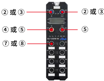
IO-Link 主站
